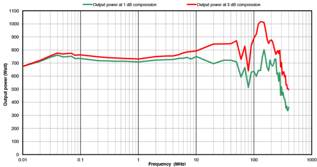
DR600 POWER AMPLIFIER 600W / 10 KHz - 400MHz
