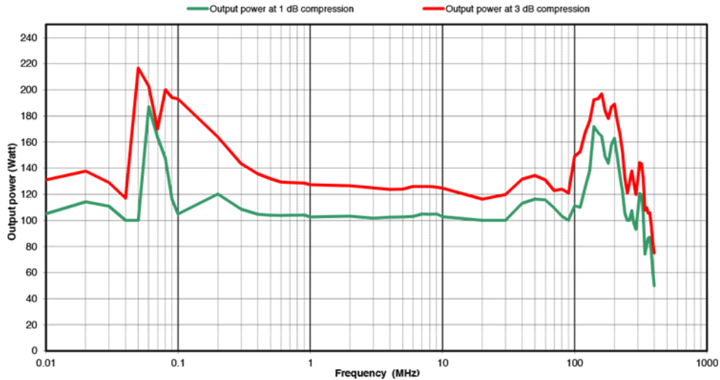
DR110 POWER AMPLIFIER 110W / 10 KHz - 400MHz
