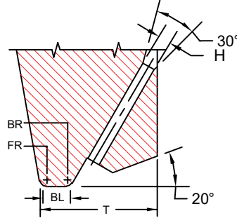
55°-60° Hole Angle
