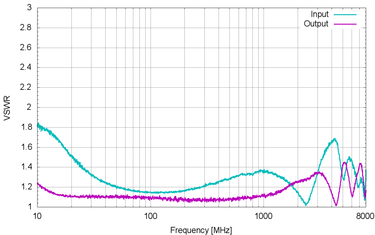
Eingangsanpassung, Ausgangsanpassung / Input Match, Output Match
